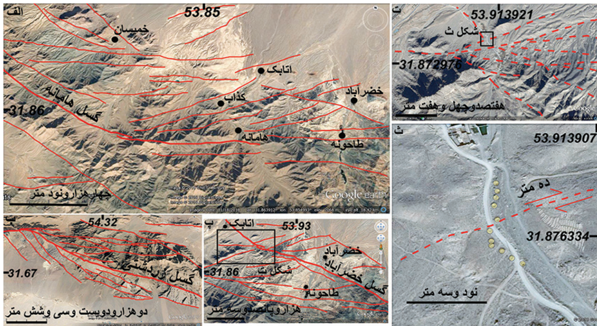
شکل ۶. تصویر ماهواره‌ای از الف. گسل هامانه. ب. گسل زردشتی در جنوب یزد. پ. اثر گسل شمال باختری خضرآباد. ت. ترسیم گسل‌های پویا در خاور خضرآباد. ث. جدایش راست بر ۱۰ متری قنات‌ها در راستای گسل خضرآباد.
