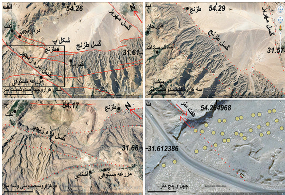
شکل ۹. الف. تصویری از موقعیت گسل‌های مهریز، طرنج و دره زنجیر. ب. گسل طرنج راستای شمال باختری دارد و برش آبرفت‌های کواترنری در مسیر آن دیده می‌شود. پ. اثر گسل شمالی-جنوبی دره زنجیر که از جنوب تفت تا حوالی طزر جان گسترش دارد. ت. جدایش راست بر ۷ متری قنات‌ها در راستای گسل طرنج.
