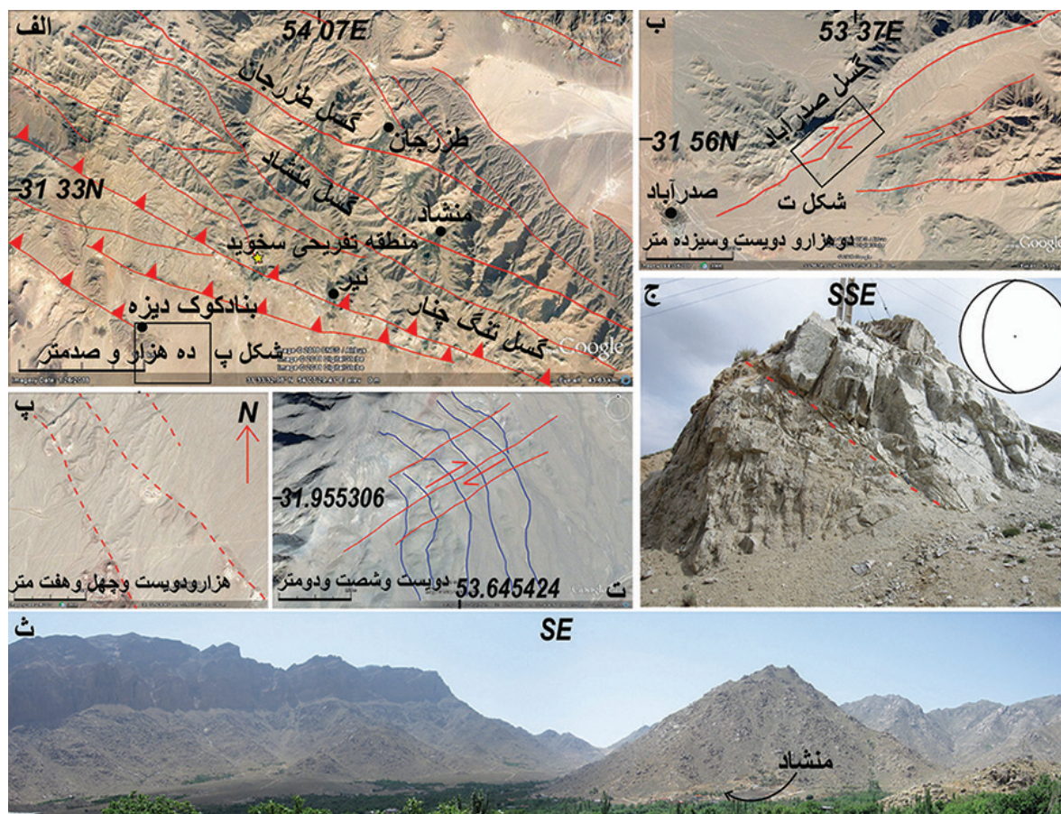
شکل ۵. الف. تصویر ماهواره‌ای از گسل‌های طزر جان، منشاد و تنگ چنار. ب. گسل راست‌الغز راست بر صدرآباد. پ. حیطه مشخص شده در تصویر الف در مقیاس بزرگتر و اثر گسلش در مخروط افکنه‌های آبرفتی. ت. جدایش راست بر آبراهه‌ها در راستای گسل صدرآباد. ث. گسلی پویا در مرز کوه و دشت که از مجاورت منشاد می‌گذرد. ج. گسل اندازه‌گیری شده در منطقه تفریحی زمستانی سخوید.
