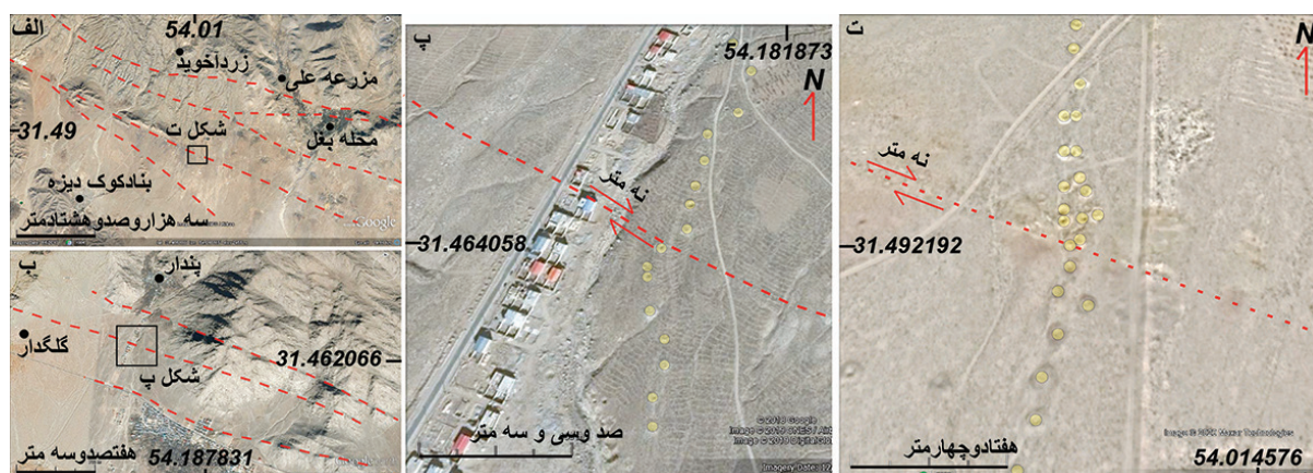
شکل ۸. الف. اثر گسل‌ها در آبرفت‌های کواترنری در جنوب زردآخوید. ب. عبور یگ گسل با راستای شمال باختری از جنوب پندار و تبیین موقعیت ایستگاههایی که جا به جایی قنات‌ها در راستای گسل را نشان می‌دهند. پ. جدایش راست بر ۹ متری قنات‌ها در جنوب پندار. ت. جدایش راست بر ۹ متری قنات‌ها در جنوب زردآخوید.
