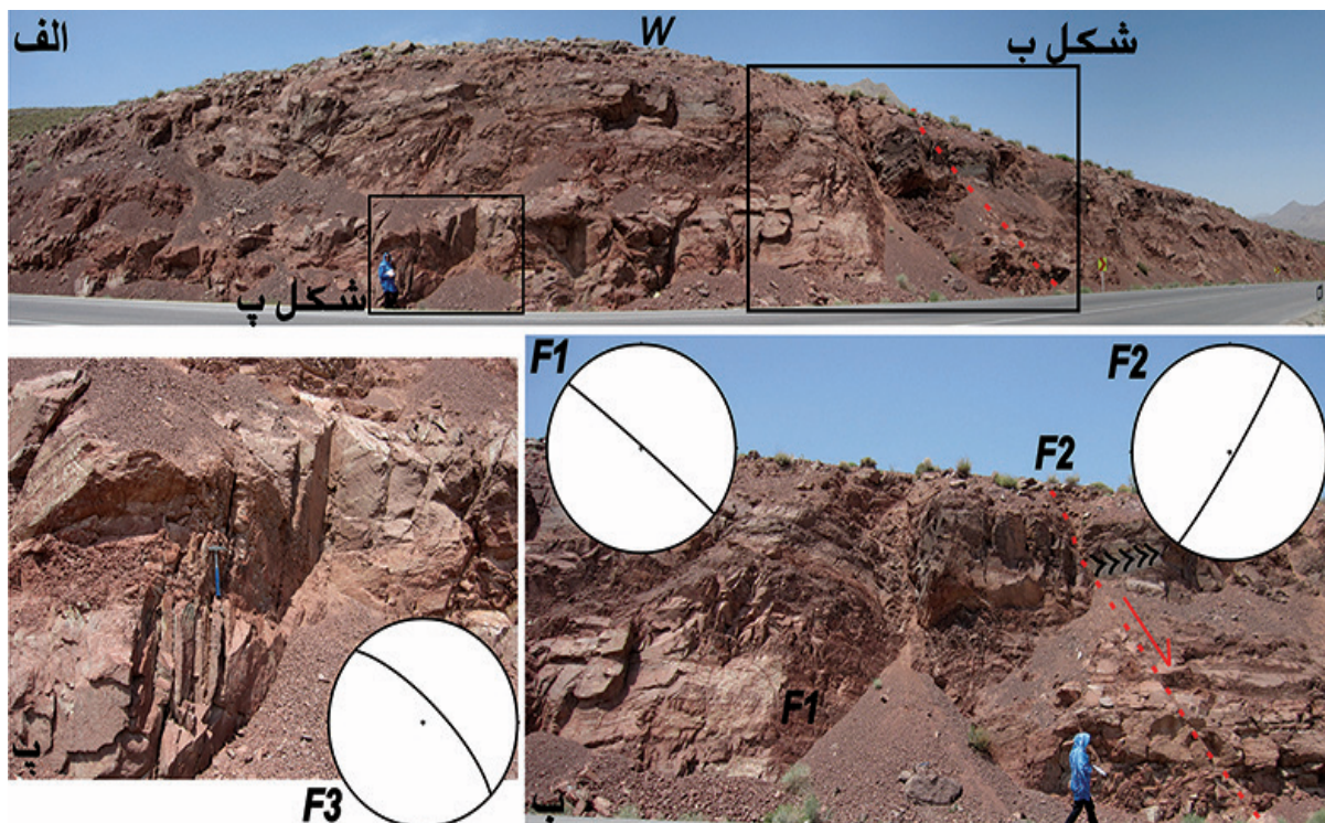
شکل ۱۵. الف. پروندگی از گسلش در ماسه سنگ قرمز گردنه علی آباد. ب. نمود نزدیک از حیطه متمایز شده در تصویر الف و صفحه‌های گسلی عادی پرشیب اندازه گیری شده. یک ساختار پرمماند در گوشه سمت راست گسل F2 دیده می‌شود. پ. جلوه‌ای بارز از محدوده معین شده به پیوست هندسه گسل برداشت شده.
