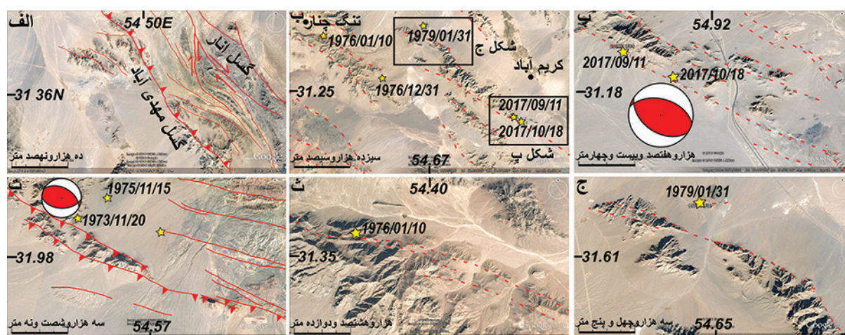
شکل ۳. الف. گسل راندگی مهدی آباد و گسل راستالغز راست بر انار. ب. نمایش موقعیت رومرکز پنج زمین لرزه در پهنه گسل تنگ چنار. داده های تکمیلی در جدول ۱ ارائه شده است. پ. گسلی در جنوب کریم آباد که رومرکز دو زمین لرزه اخیر بر روی آن قرار دارد. سازوکار کانونی زمین لرزه هیجده اکتبر ۲۰۱۷ در این تصویر مشاهده می شود. ت. رومرکز سه زمین لرزه در شمال خاور یزد. سازوکار کانونی زمین لرزه بیست نوامبر ۱۹۷۳ در شکل ارائه شده است. ث. رومرکز زمین لرزه روی داده در جنوب تنگ چنار. ج. رومرکز زلزله ای در خاور تنگ چنار و عملکرد گسلش پویا در این خطه.
