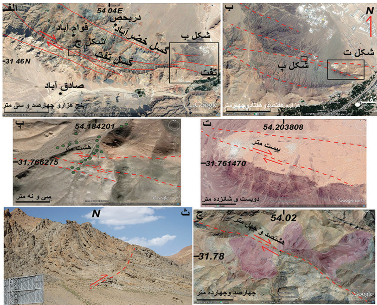
شکل ۲ الف. تصویر ماهواره‌ای از گسل‌های خضر آباد و تفت. ب. ترسیم اثر گسلش پویا در شمال تفت. پ. جدایش راست بر ۸ متری قنات‌ها در پایانه خاوری گسل تفت. ت. جدایش راست بر ۲۰ متری در آبرفت‌های کواترنری در پایانه خاوری گسل تفت. ث. چین خوردگی لایه‌های آهکی در اکناف اسلامیه. یک گسل راندگی این لایه‌های چین خورده را بریده است. ج. بر آورد ۸۴۰ متر جا به جایی راست بر در واحدهای تریاس در راستای گسل تفت.
