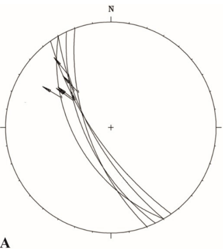
شکل ۸) ایستگاه شماره ۱۹ مجموعه دگرگونی تکاب. در قسمت A، سازوکار راستالغز راست گرد با مولفه‌ی فرعی شمال و قسمت B، خش لغز موجود در این ایستگاه گسل نمایش می‌دهد.
