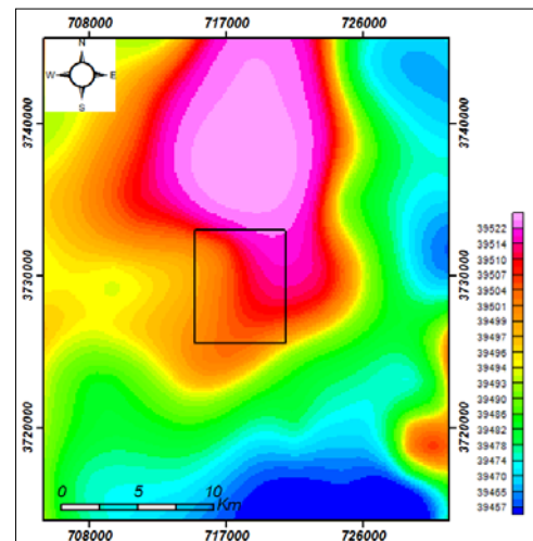
شکل ۱۰: نقشه شدت کل میدان مغناطیسی، مناطق قرمز بیانگر شدت بیشتر میدان مغناطیسی و مناطق آبی نشان دهنده شدت کم میدان است. کادر مشکی محدوده مورد مطالعه را نشان می‌دهد.
